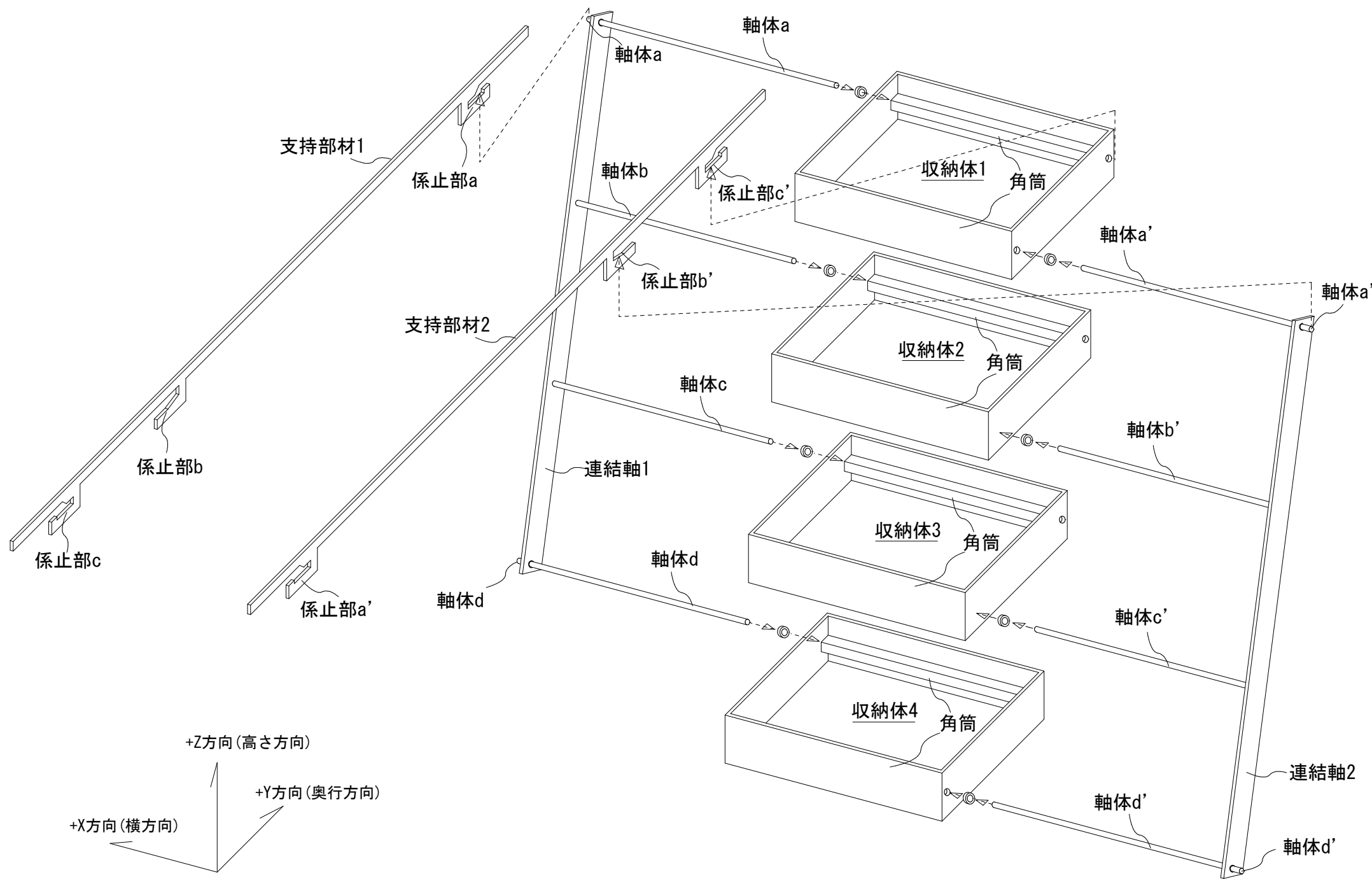
図A: 斜視図 (分解図)
