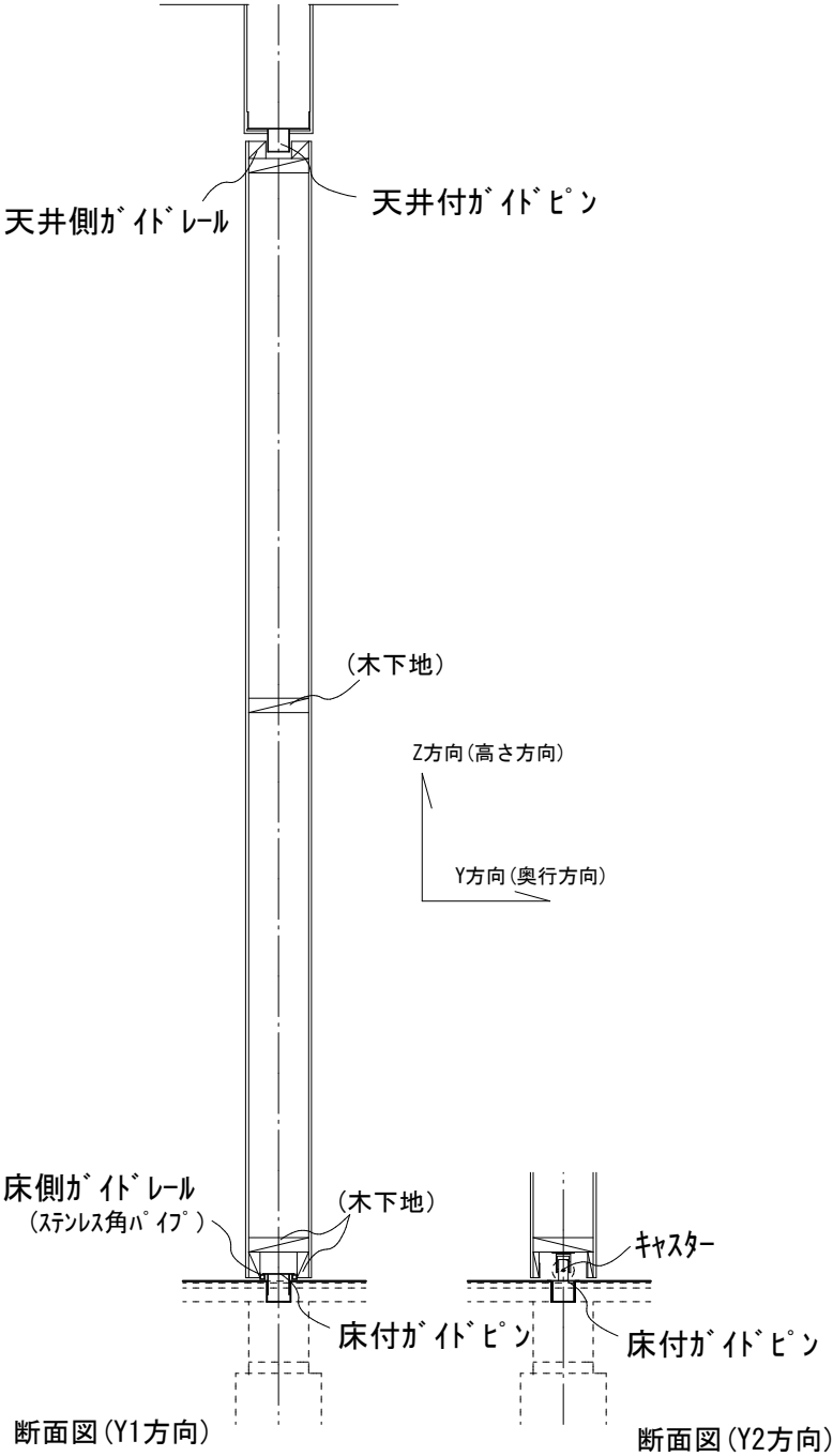
図I:断面図
