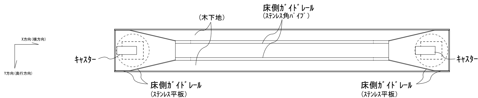
側面図(下面)
